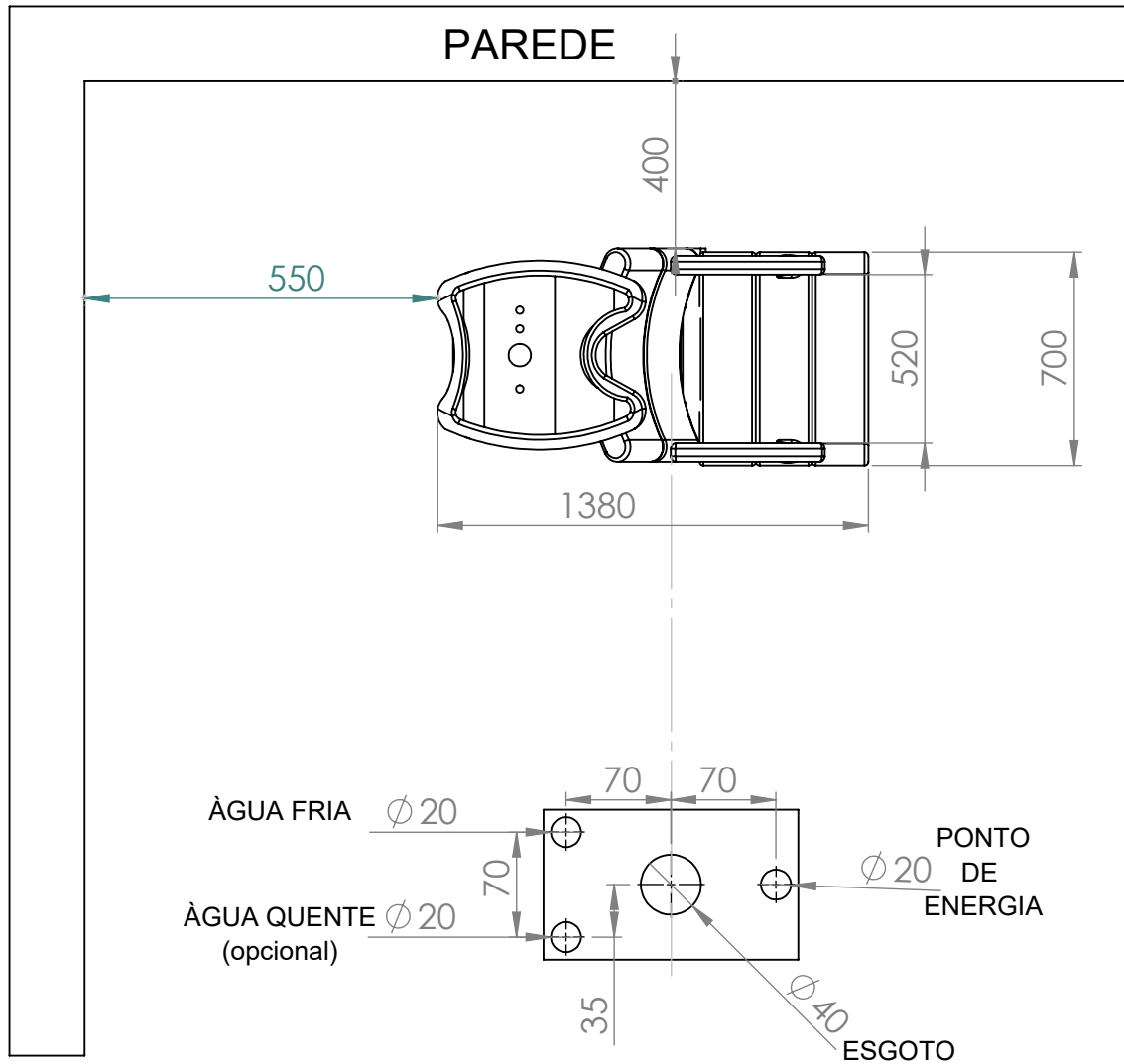
Esquema de instalação (Sob acento)
